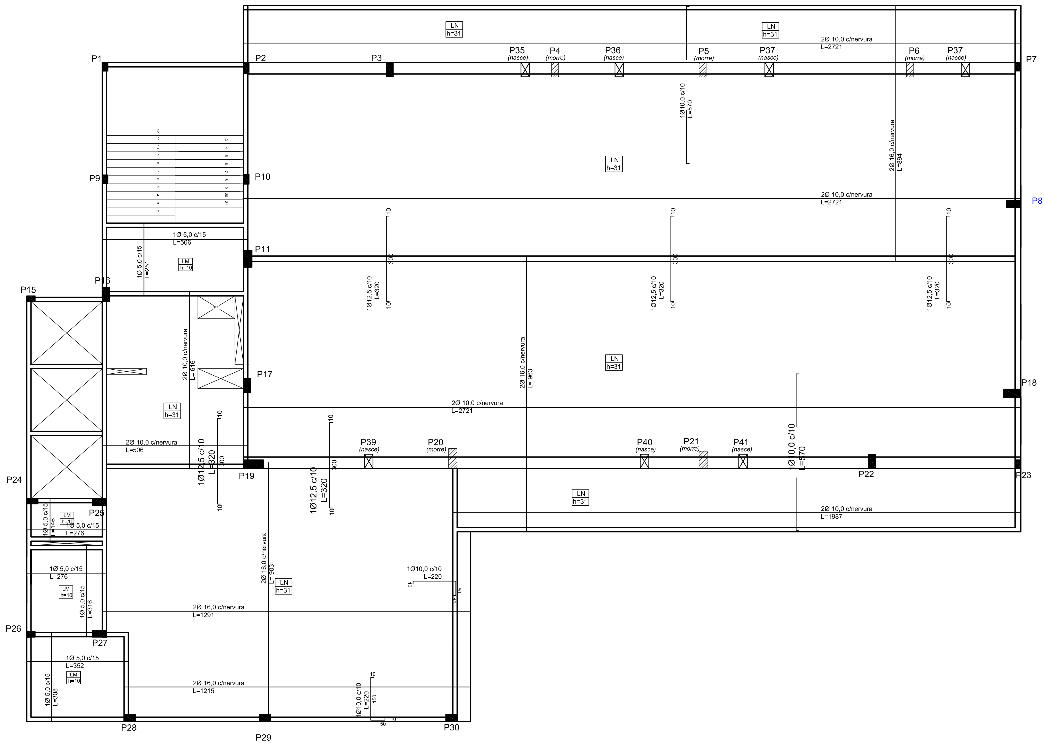
Planta de Fôrmas 5º Pavimento - Ferragem Escala 1:75
